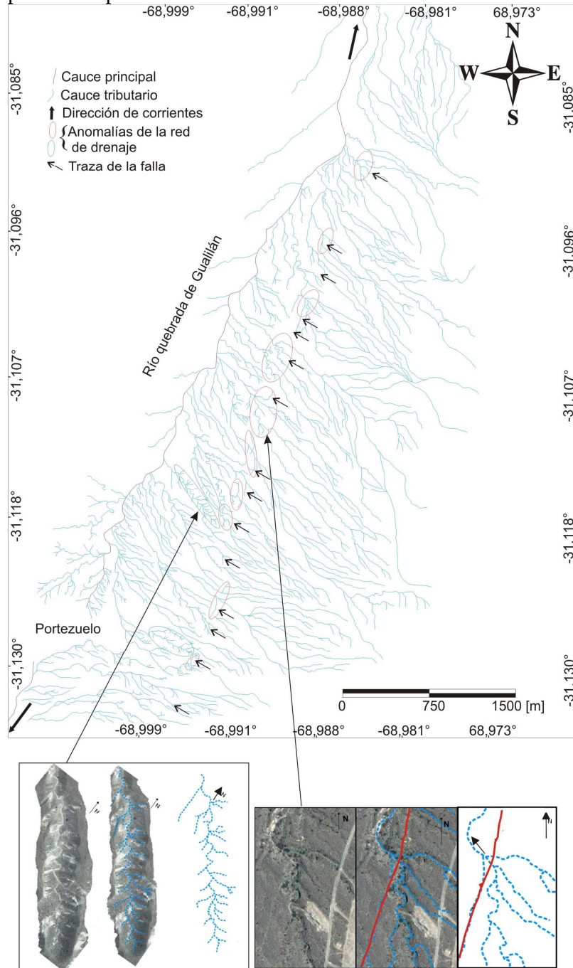
Figura 2. Anomalías de la red de drenaje en el corrimiento La Cantera
