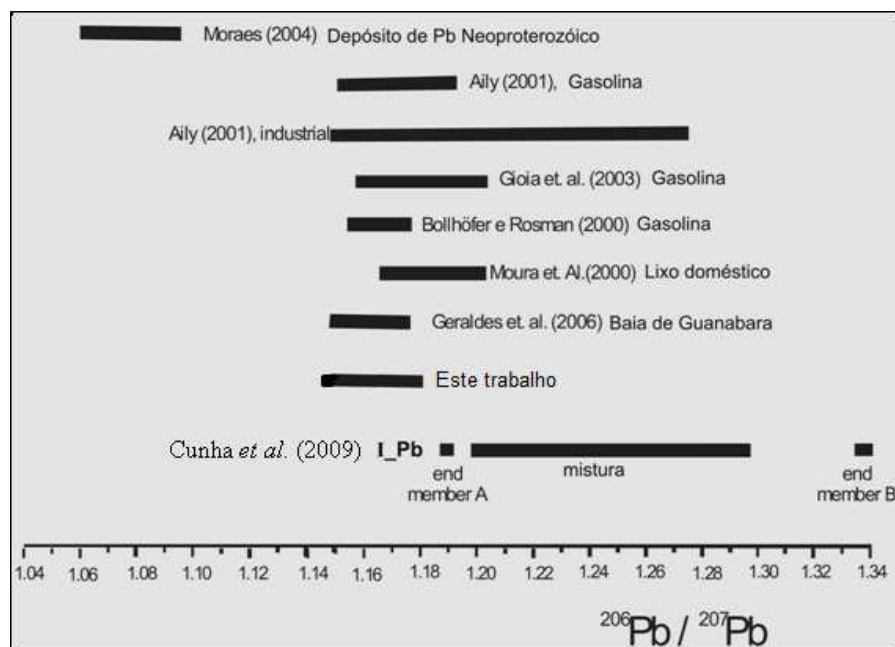
Fig.4. Razões ^{206}\text{Pb}/^{207}\text{Pb} encontradas na literatura e neste trabalho.
